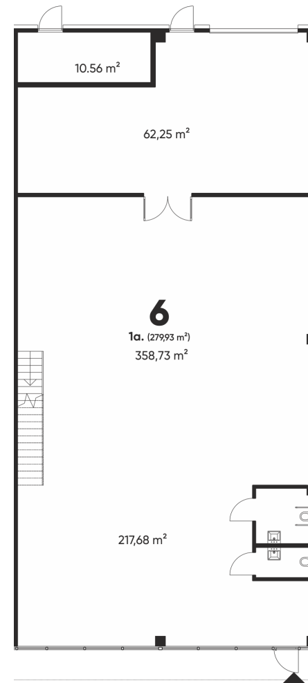
1 aukšto planas
