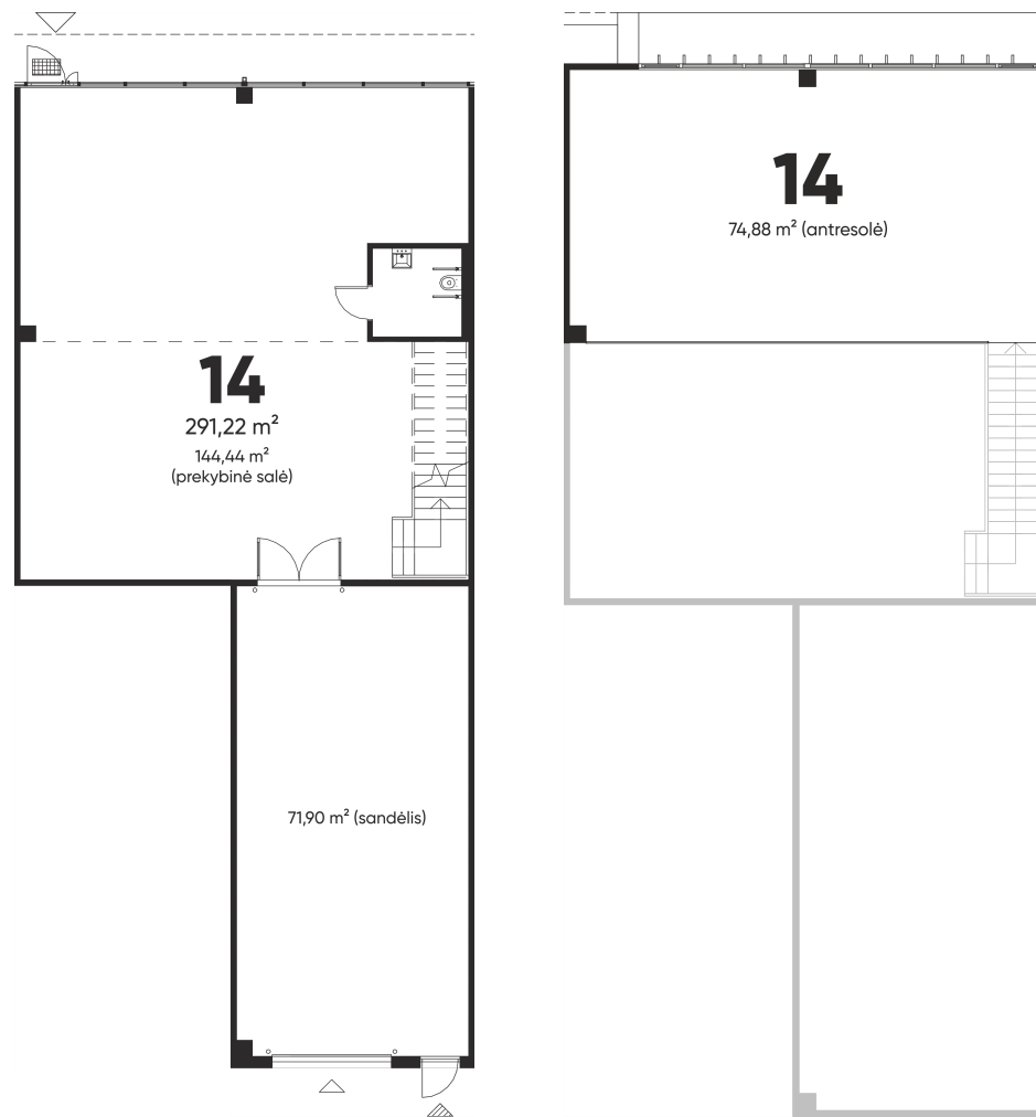
1 aukšto planas
