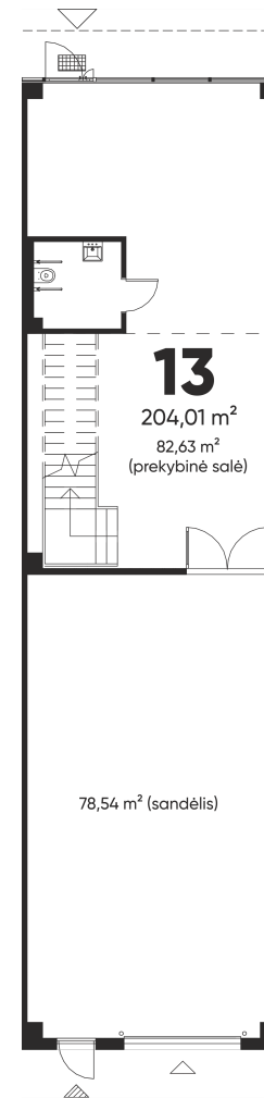
1 aukšto planas
