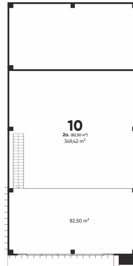
2 aukšto planas
