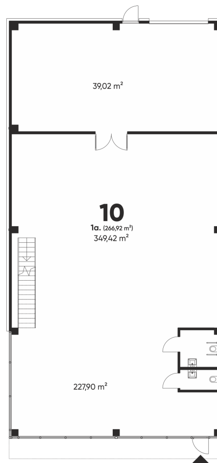
1 aukšto planas
